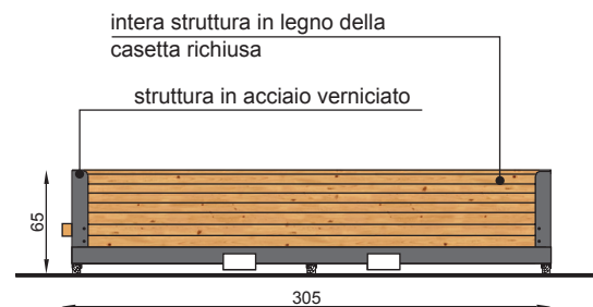
ingombro casetta richiusa
