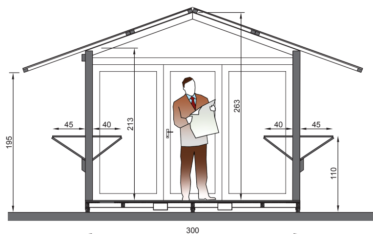
sezione frontale
