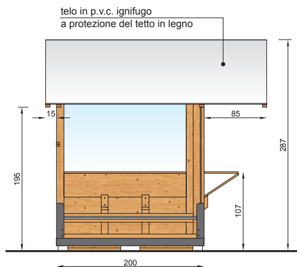
prospetto laterale
