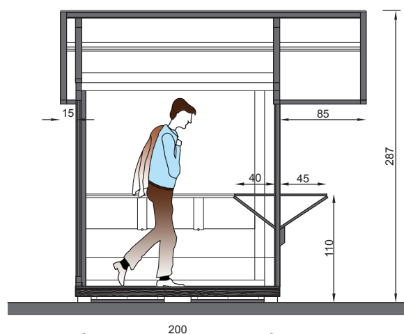
sezione laterale
