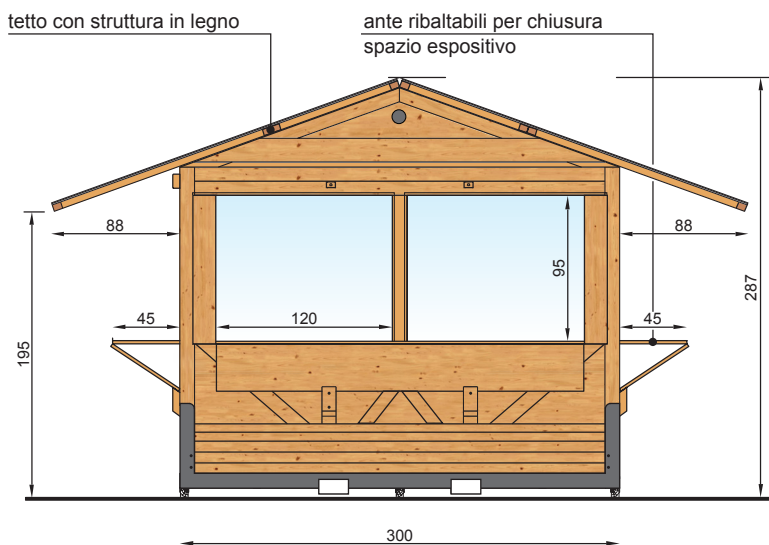
prospetto frontale
